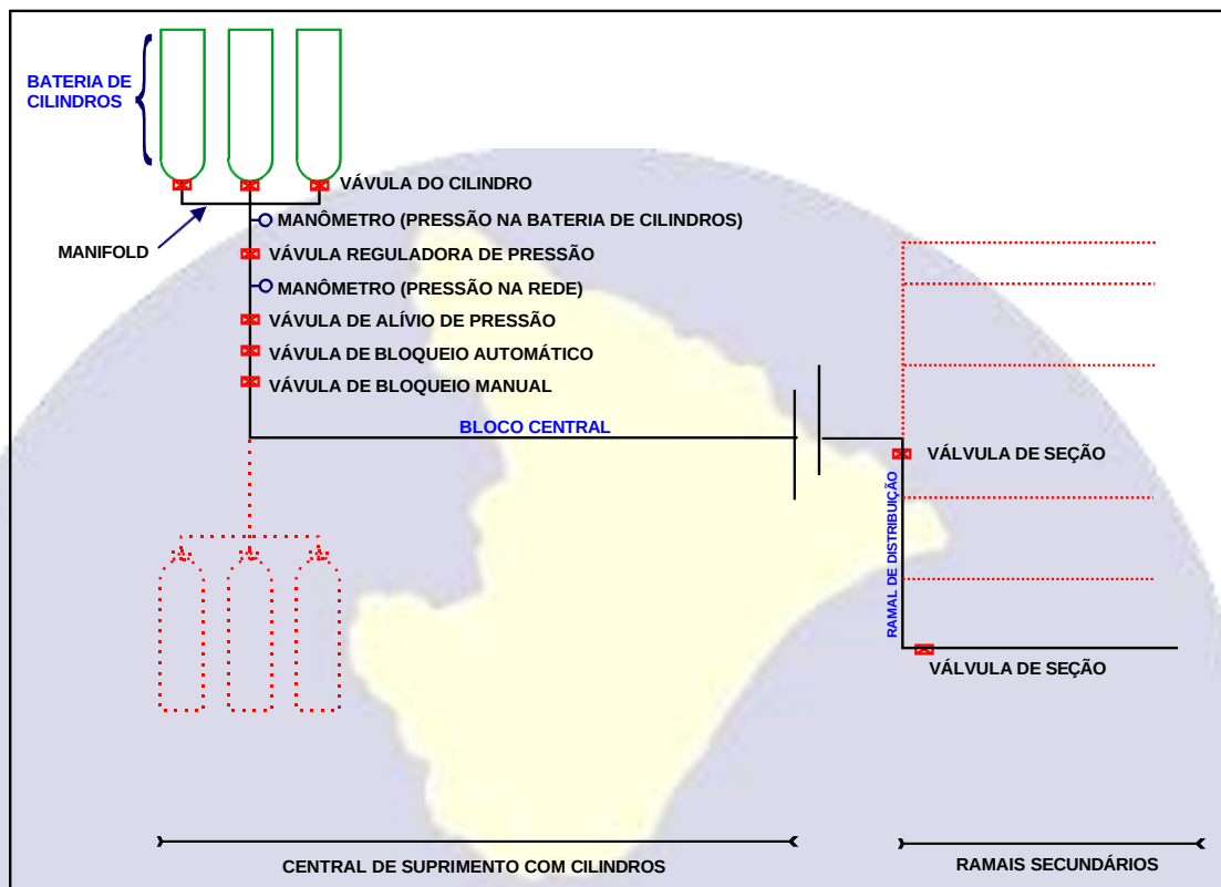
Fig 12. Central de Suprimento com Cilindros - Desenho Esquemático.
