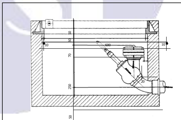
Fig 07. Hidrante de Recalque - Corte. Hidrantes Tipo Coluna
