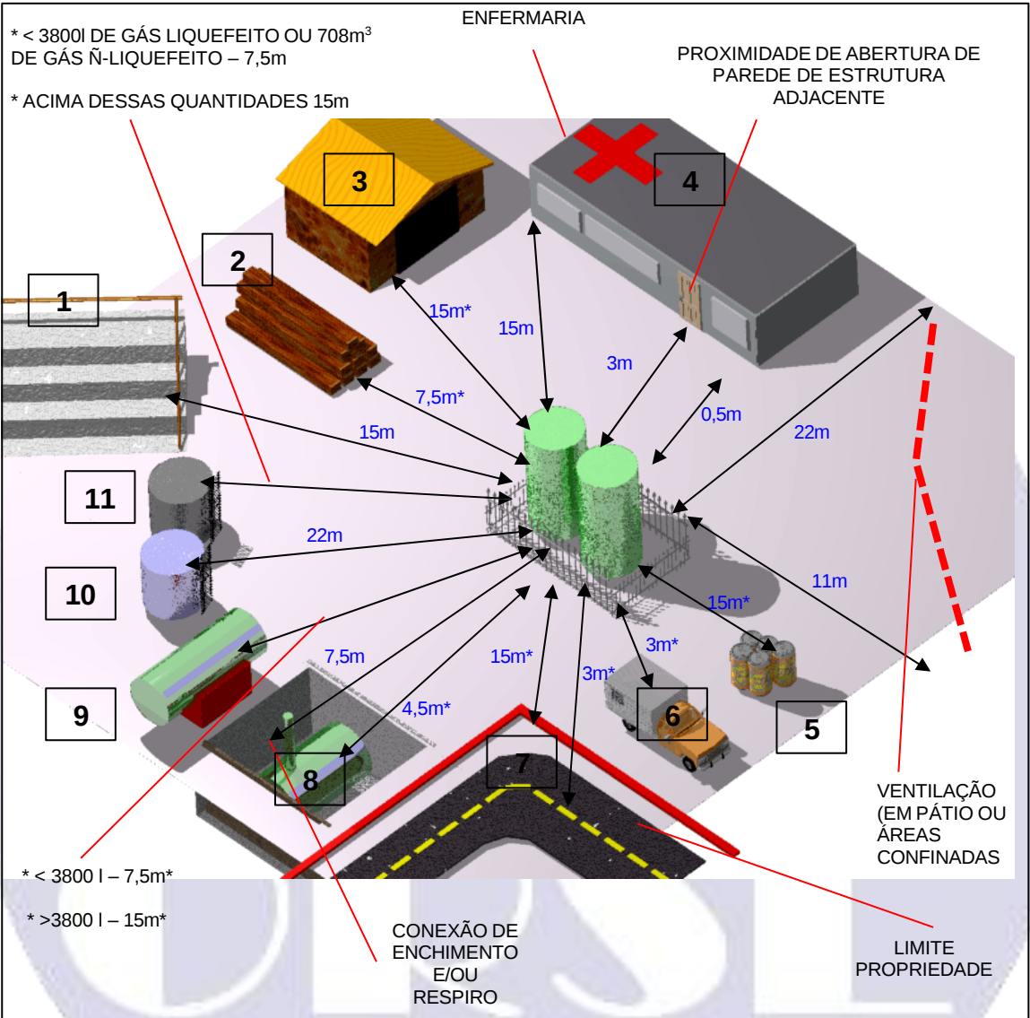
Fig 13. Distâncias mínimas entre o Sistema de Oxigênio Líquido e adjacências.
