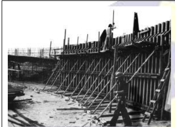
Figura 21 - Execução de Cimbramento para Formas Verticais
