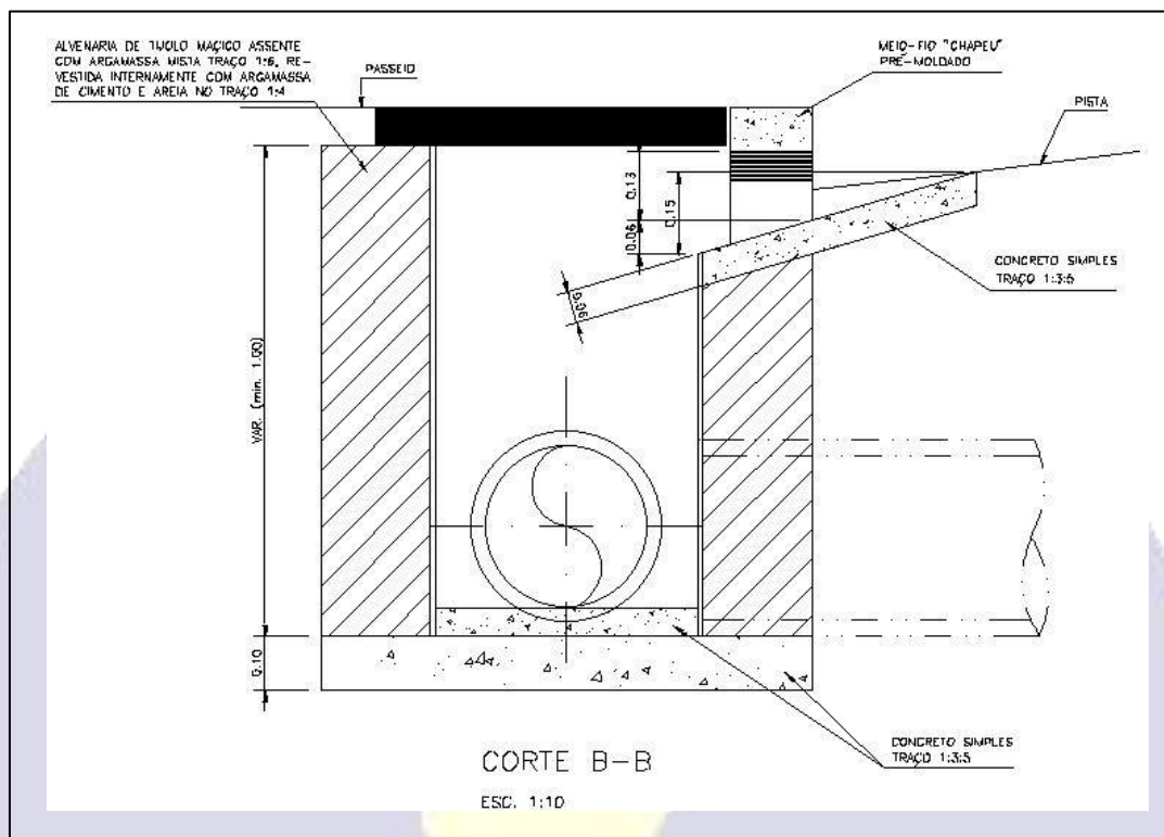
Figura 06. Boca de Lobo com Depressão - Corte BB
