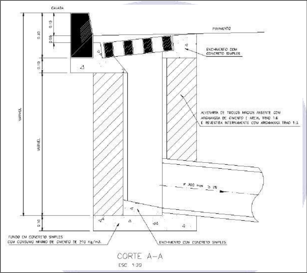
Figura 02. Boca de Lobo com Grelha - Corte AA
