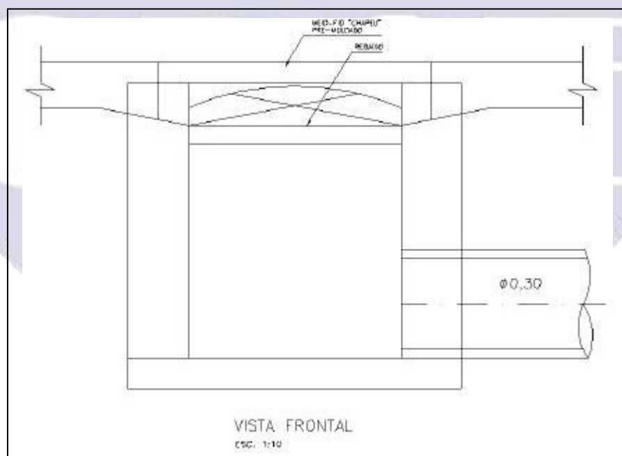
Figura 07. Boca de Lobo com Depressão – Vista Frontal
