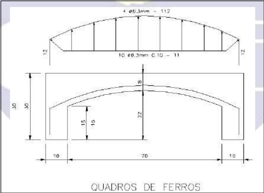
Figura 08. Meio-Fio “Chapéu” - Armação - (Dimensões em cm, Bitolas em mm)
