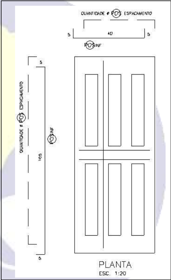
Figura 04. Grelha / Armação - Planta
