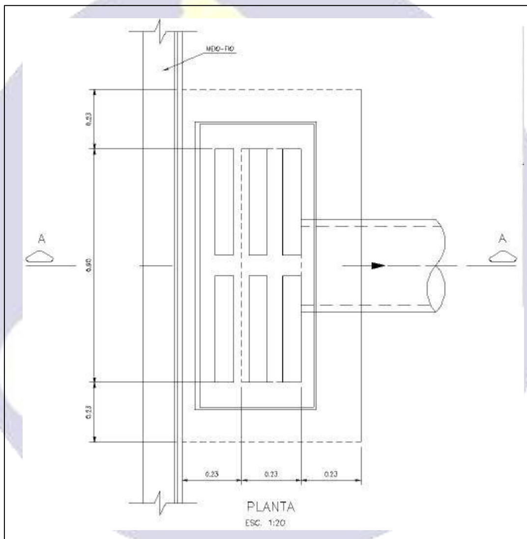
Figura 01. Boca de Lobo com Grelha - Planta
