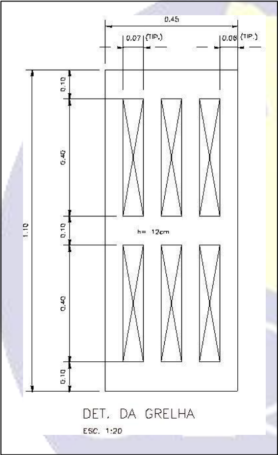
Figura 03. Grelha / Armação - Detalhes
