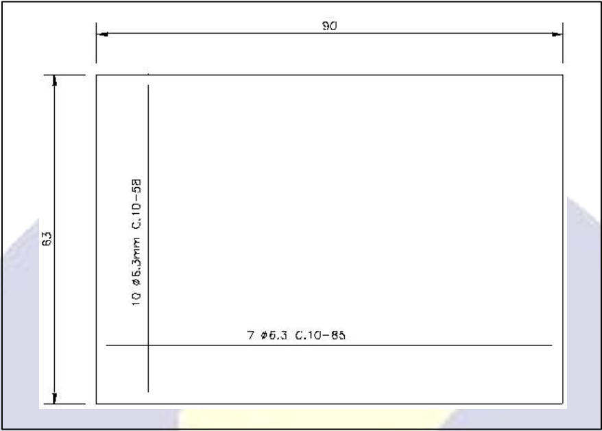
Figura 08. Tampa de Boca de Lobo (Dimensões em cm, Bitolas em mm)
