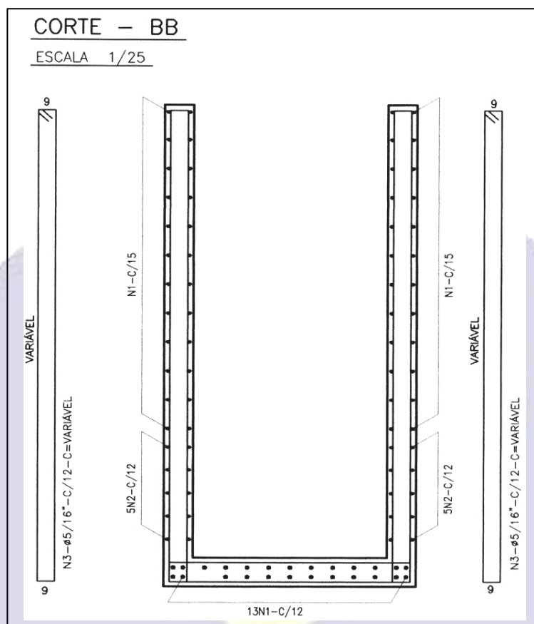
Fig 05. Corte BB
