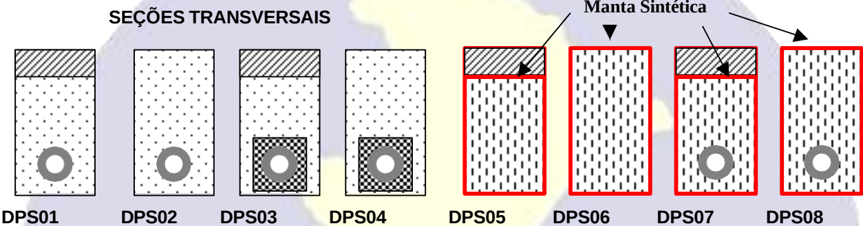
Figura 01. Drenos longitudinais profundos para cortes em solo - Terminologia DNER
