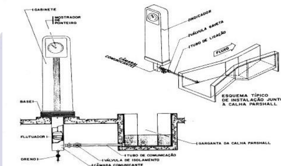
Figura 01. Calha Parshall e Indicador de Vazão.
