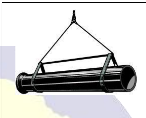
Fig. 02. Movimentação com utilização de cintas e "balancim"
