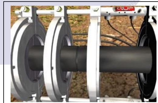
Fig. 19 - Em seguida, deverá ser verificado o perfeito alinhamento dos dois tubos.
