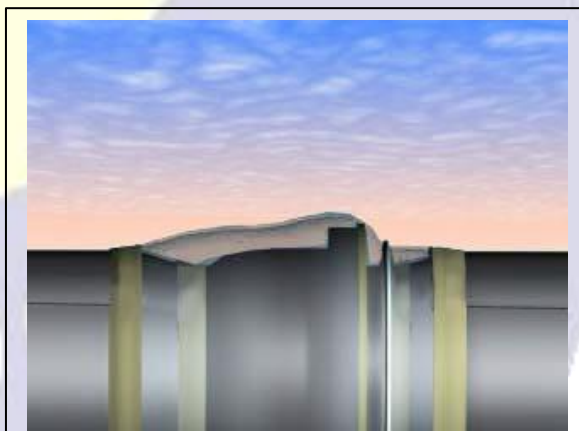
Fig. 15 - A manta deverá ser dobrada e esticada ao máximo, ou seja, acompanhando o perfil da bolsa e recobrimdo a manta do corpo do tubo. Nesta região, a dobra de rebatimento também deverá ficar na geratriz superior.
