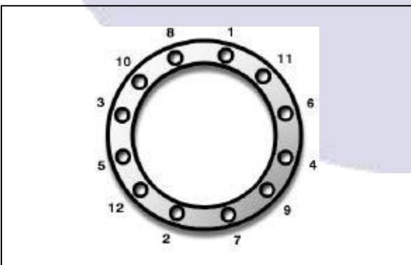
Fig. 08- Sequência de aperto das porcas
