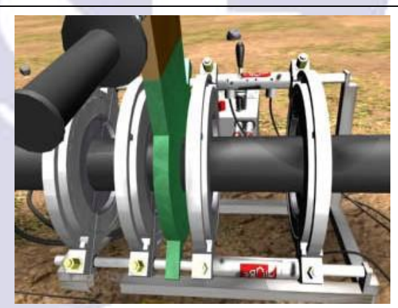
Fig. 24 - Formado o cordão, a pressão de solda e o contato da placa com os tubos deverão ser mantidos pelo tempo recomendado pelo fabricante do equipamento.
