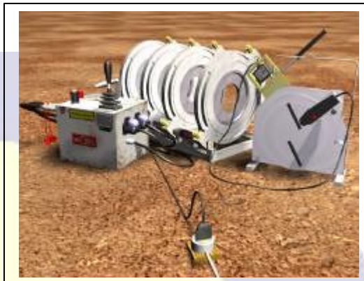
Fig. 17 - Equipamento de solda de topo
