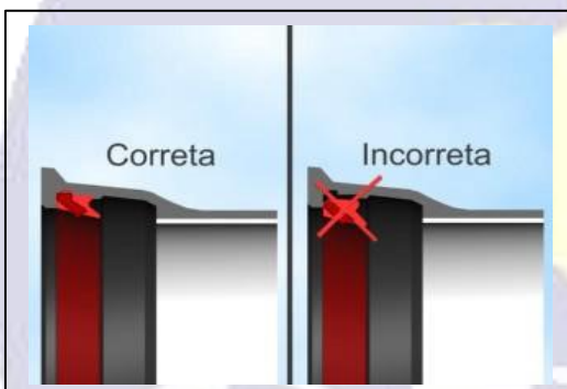
Fig. 03 - Verificação da colocação do anel de borracha
