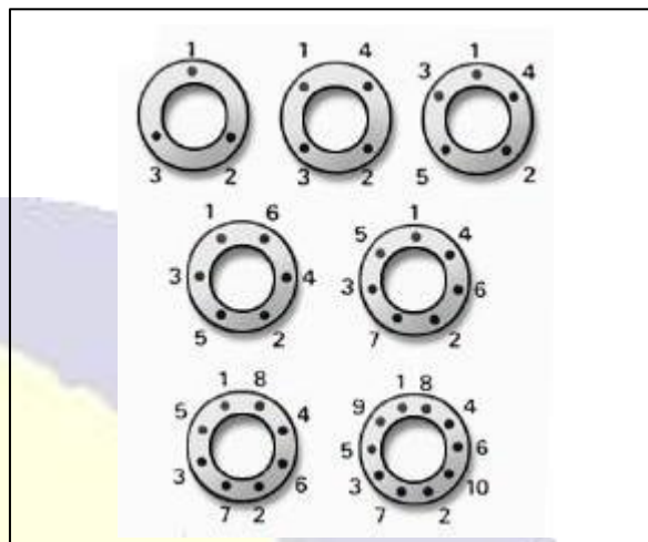
Fig. 08 - Deverá ser seguida a sequência de aperto de parafusos indicada acima.
