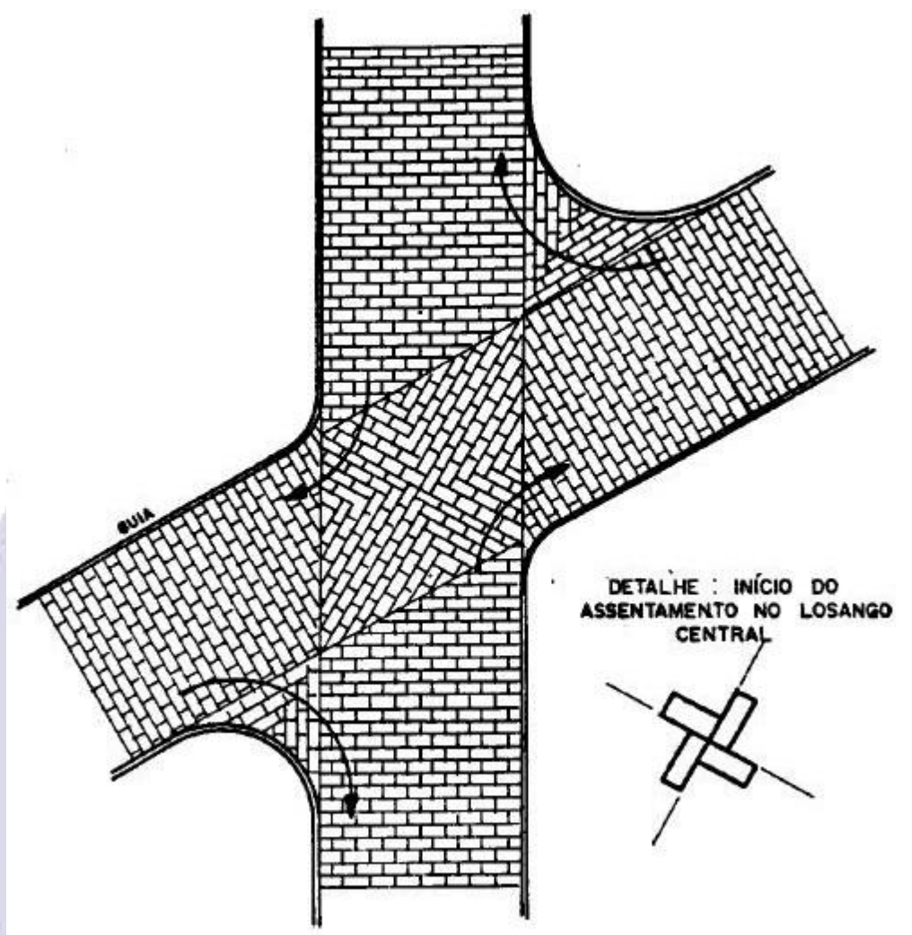
Figura 07. Cruzamento Esconso de 2 Vias Principais ou Secundárias
