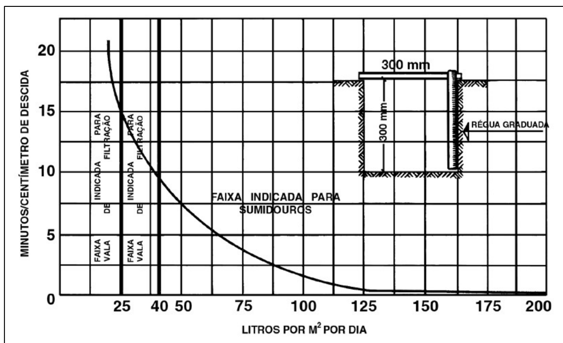
Figura 05. Gráfico para cálculo do coeficiente de percolação
