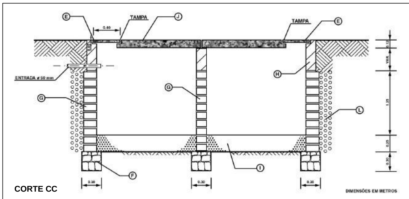
Figura 08. Sumidouro – Corte CC
