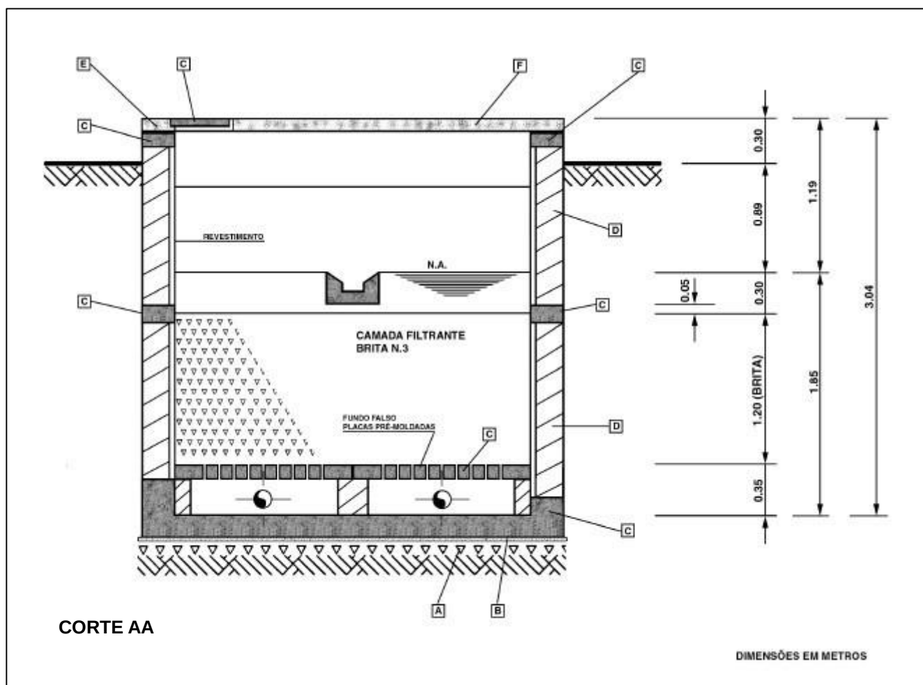
Figura 03. Filtro Anaeróbico padrão CEHOP para 50 casas – Corte AA
