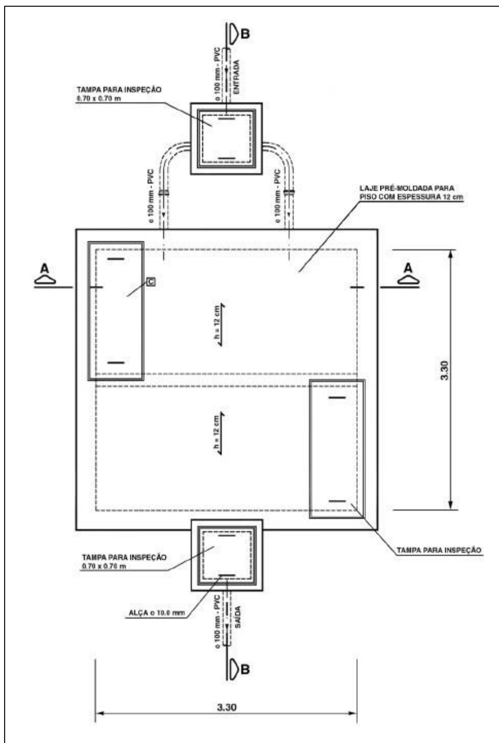
Figura 01. Filtro Anaeróbio padrão CEHOP para 50 casas – Vista Superior
