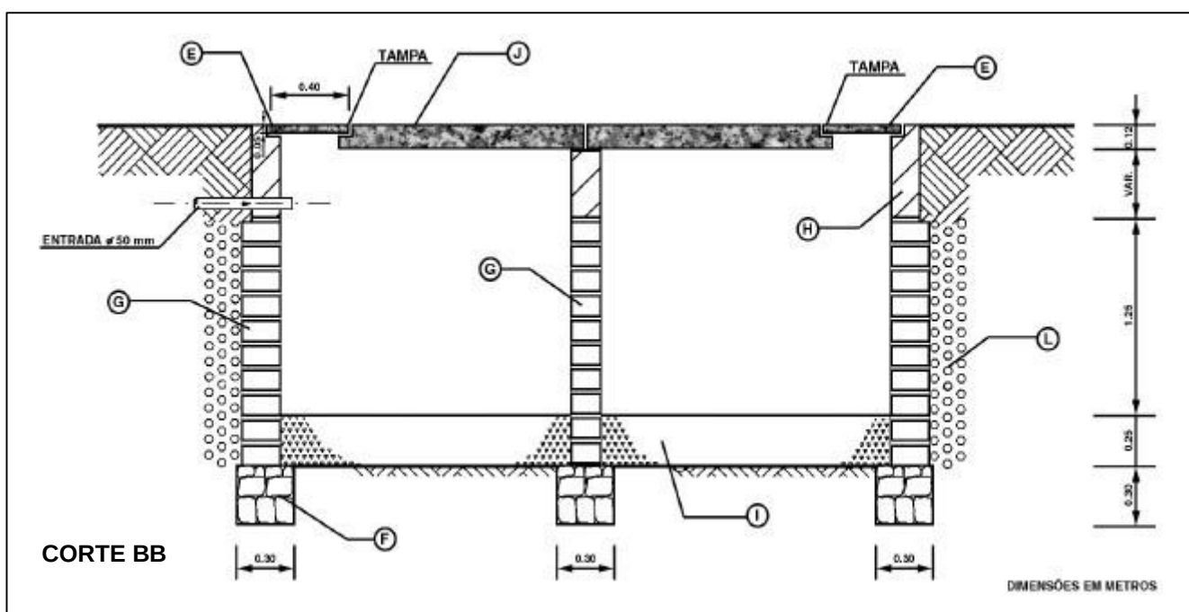
Figura 07. Sumidouro – Corte BB
