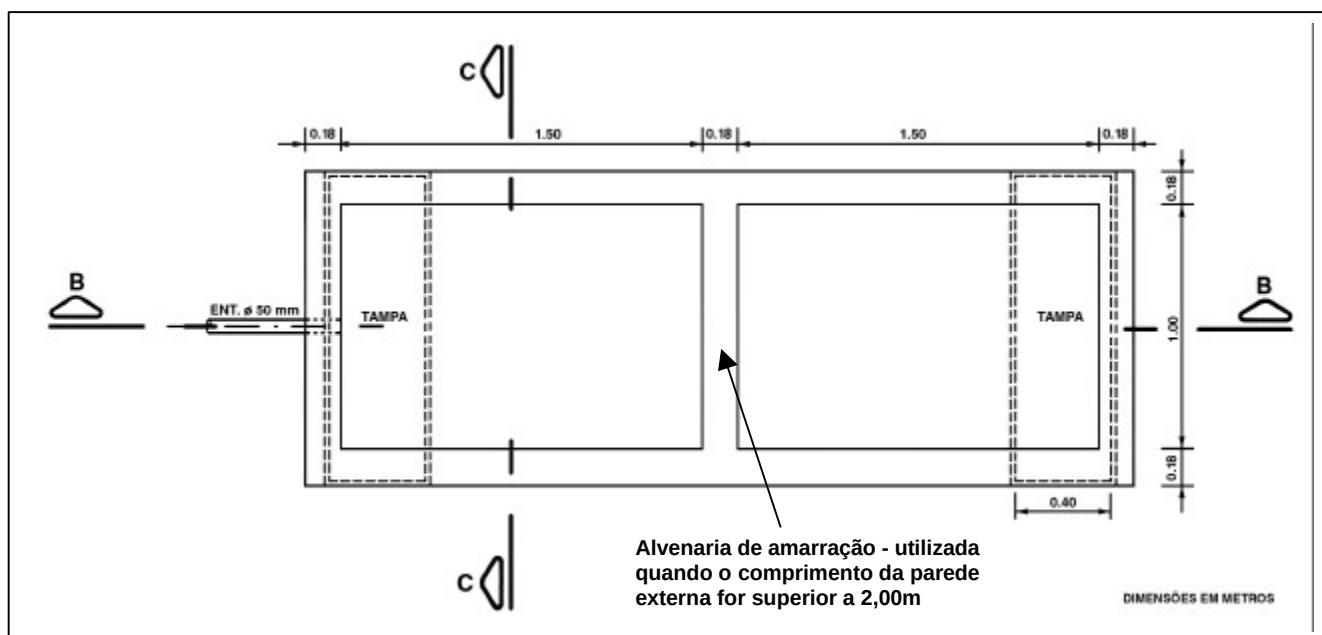
Figura 06. Sumidouro – Planta Baixa
