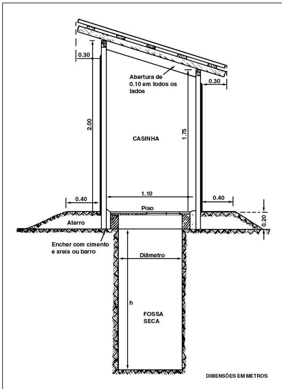
Figura 01 - Fossa Seca - Corte
