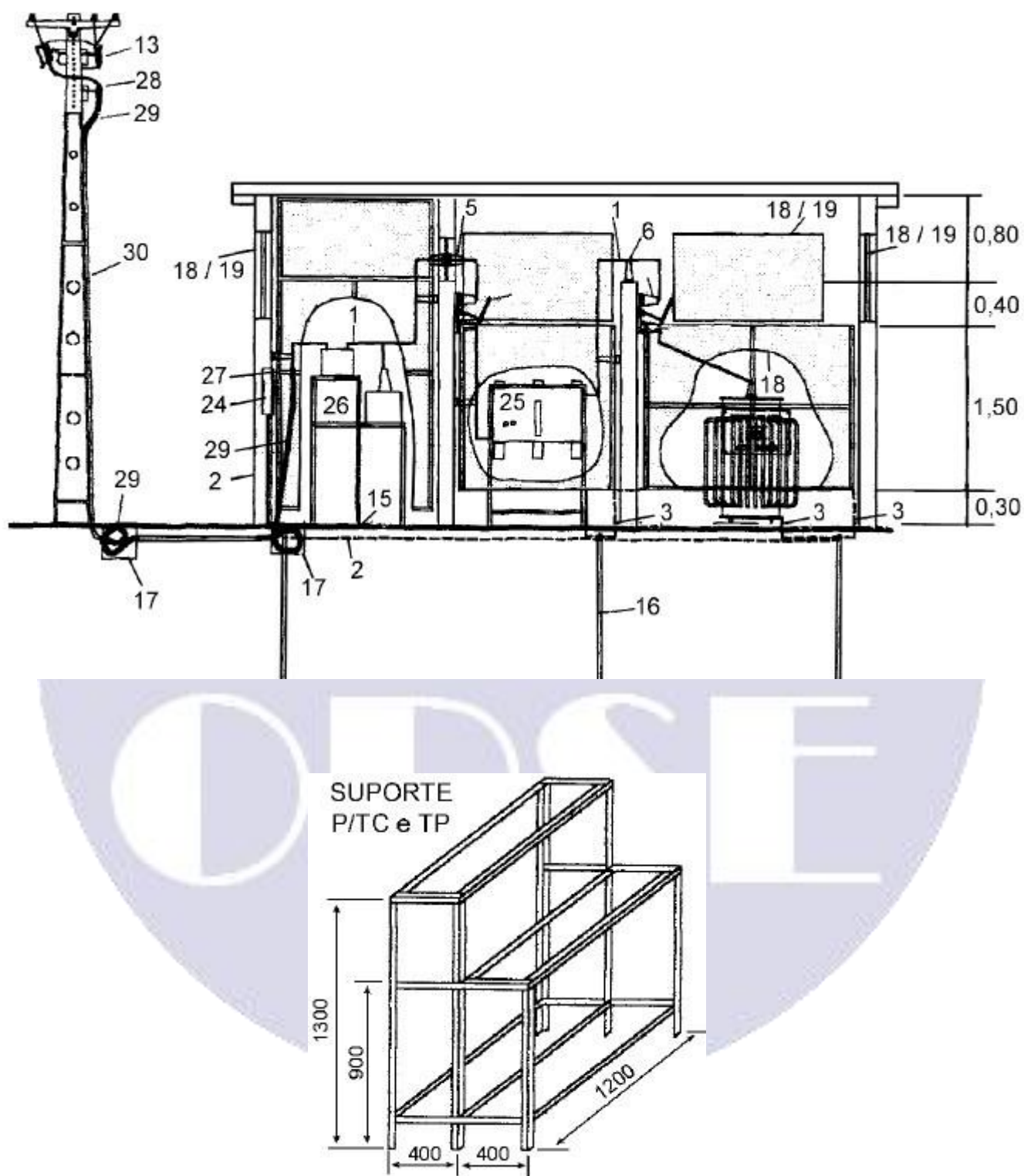
Figura 03. Subestação Transformadora Abrigada, Entrada Subterrânea, Medição AT - CORTE A – A
