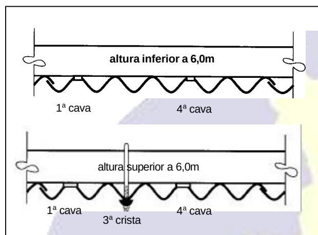
Figura 03. Fixação de telhas centrais
