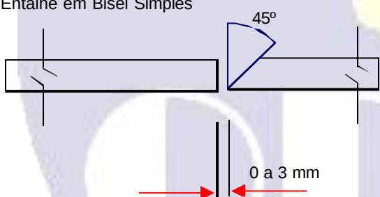
Entalhe em Bisel Simples
