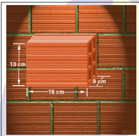
Figura 01. Alvenaria singela com blocos cerâmicos 06 furos
