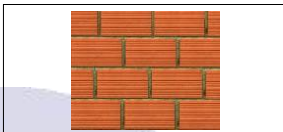
Figura 30. Junta Amarrada
