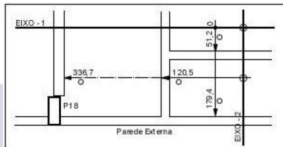
Figura 39. Sistema de cotas da planta de marcação
