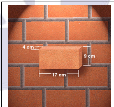
Figura 05. Alvenaria com tijolos cerâmicos maciços a facão
