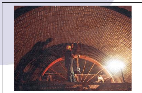
Figura 28. Revestimento Básico em Forno de Cimento
