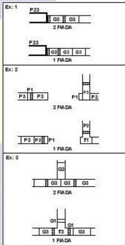
Figura 42. Juntas verticais
