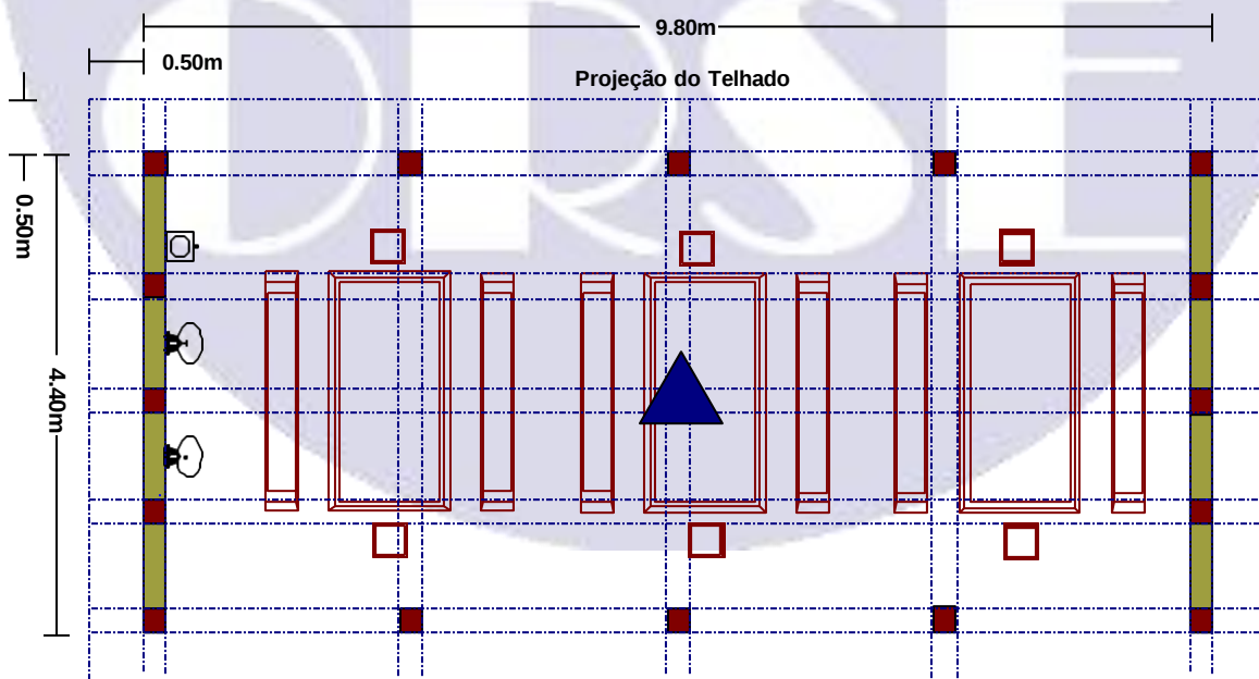
Planta da Cobertura
